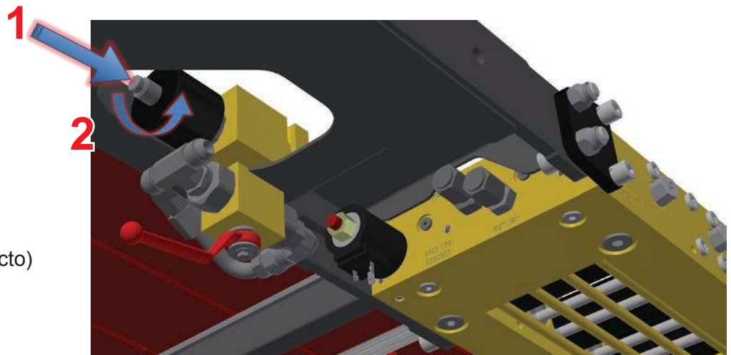
Anulación manual – Válvula de control (Solenoide)
