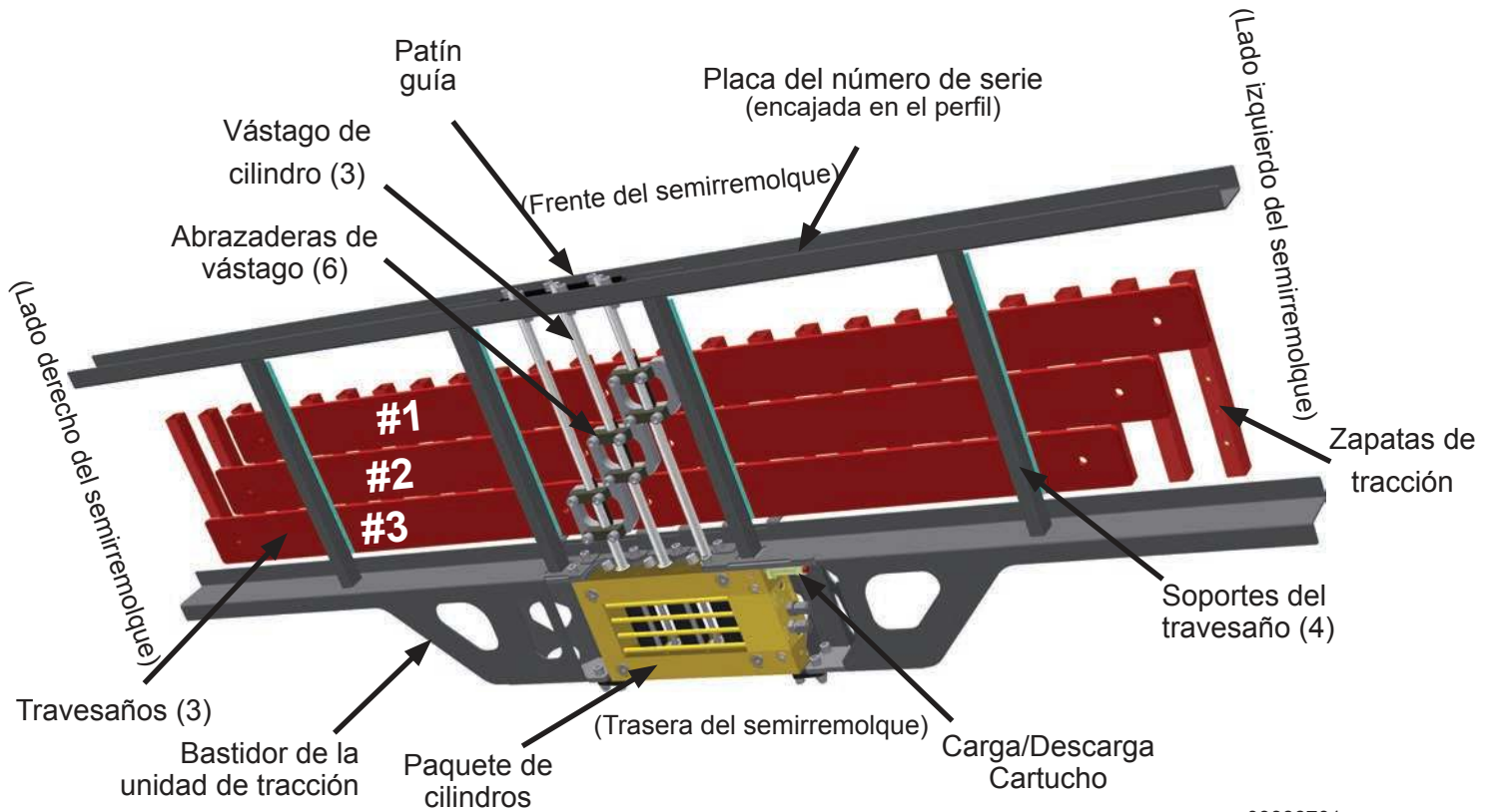
Vista desde debajo del semirremolque
